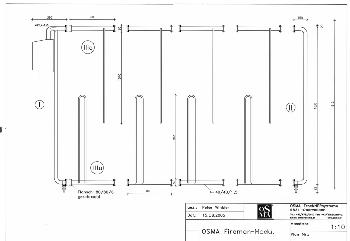
Detailskizze
